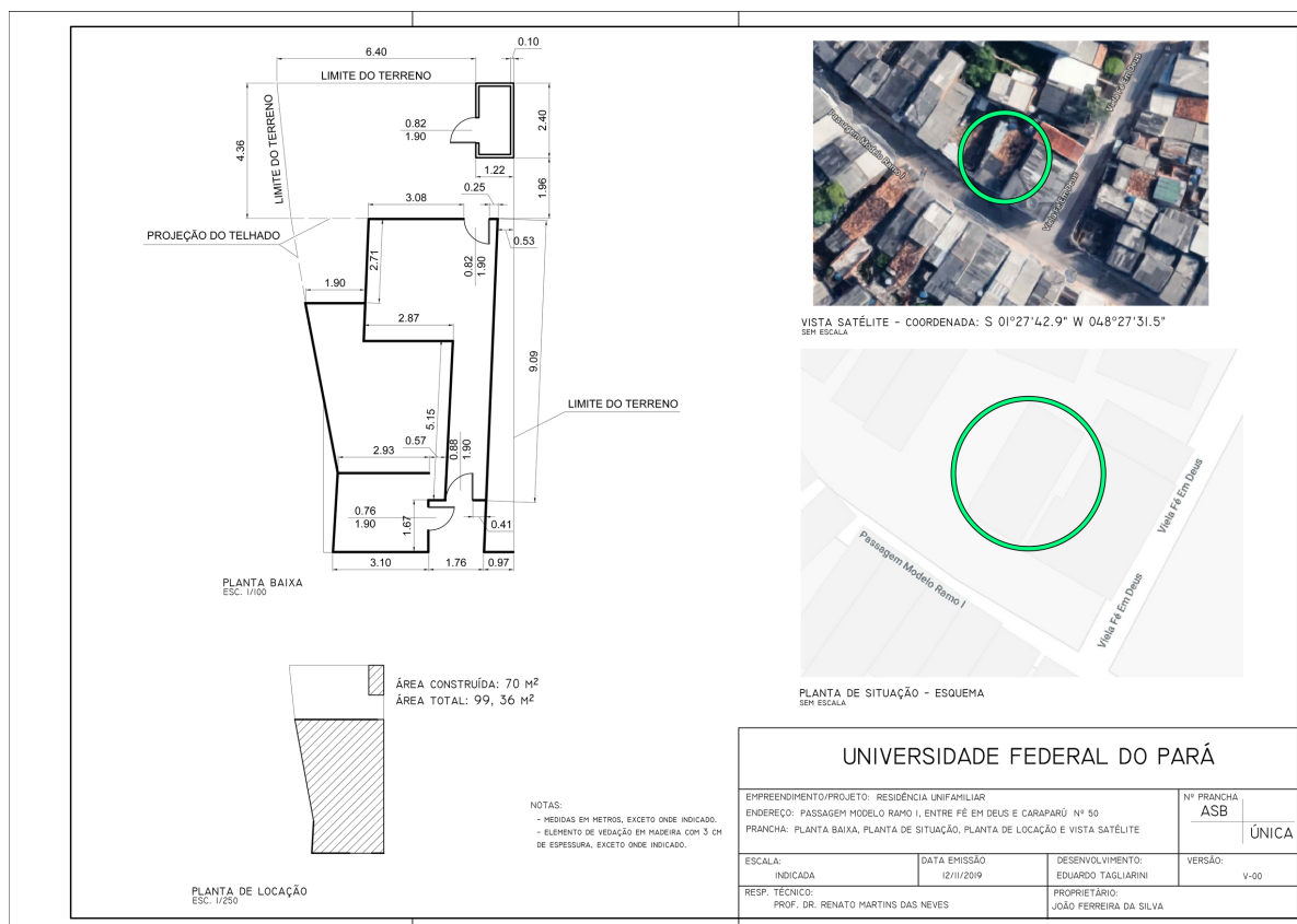
Planta Baixa I Residencial J.F.Silva, 2019.
