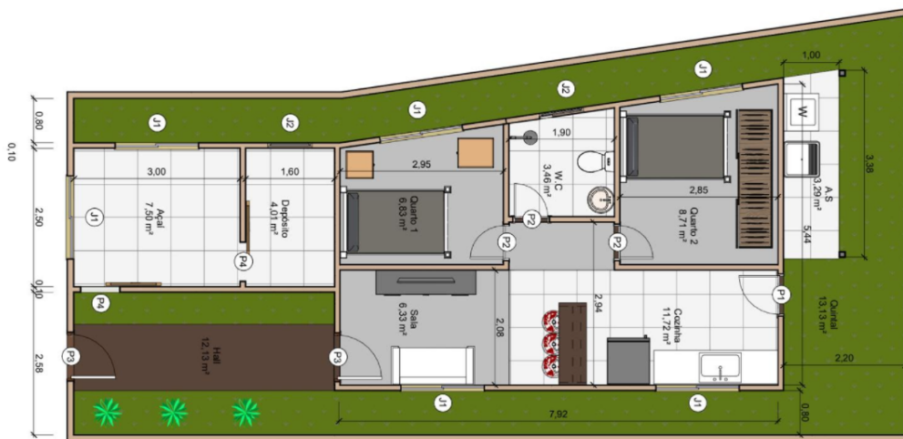
Planta Baixa IV Residencial J.F.S
