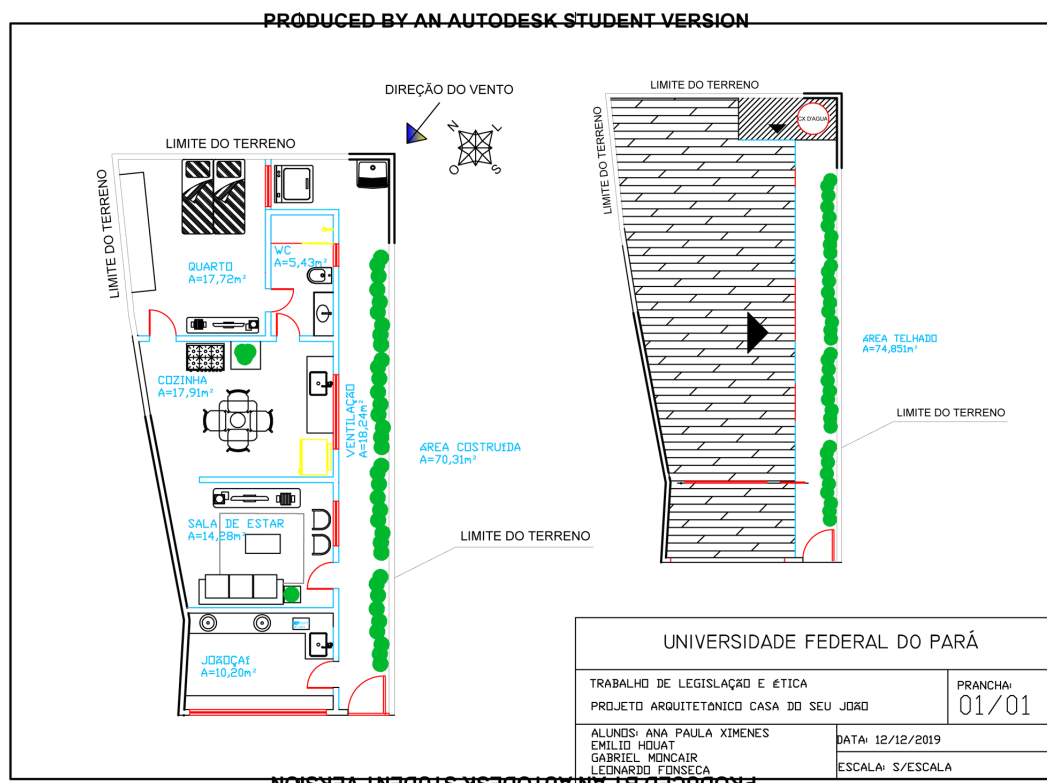
Planta Baixa II Residencial J.F.S, 2019.
